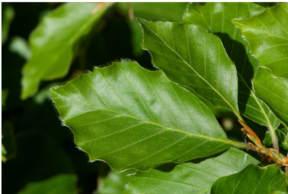
Буква - Fagus silvatica
