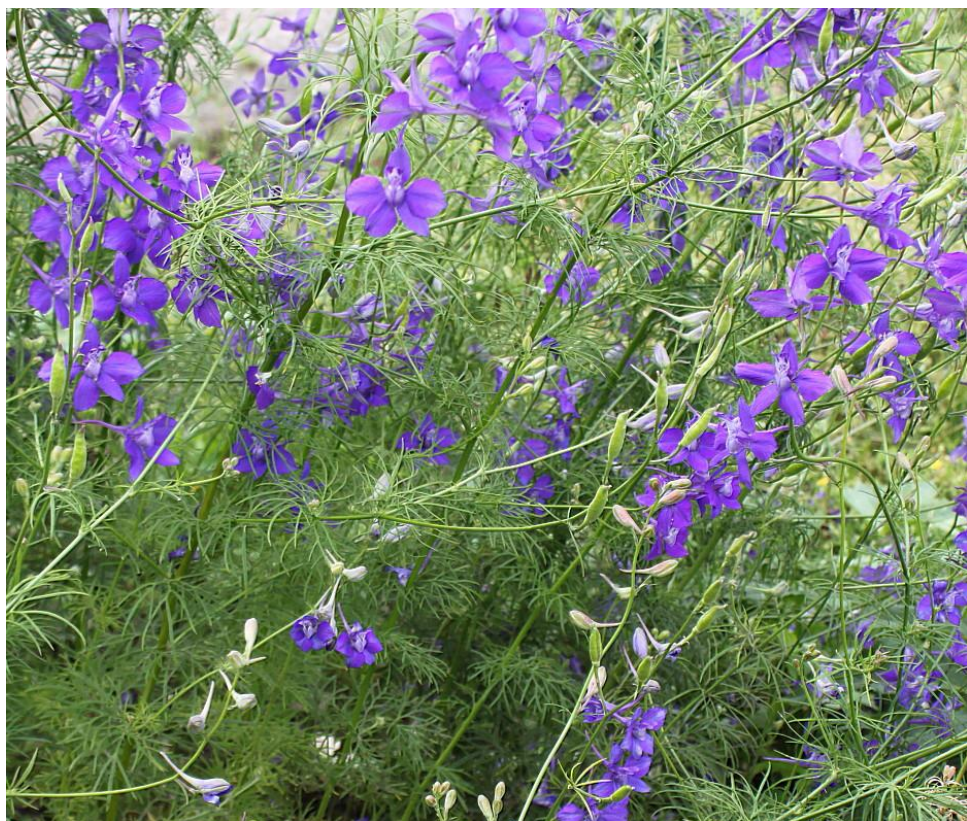
Жаворњак - Consolida regalis
