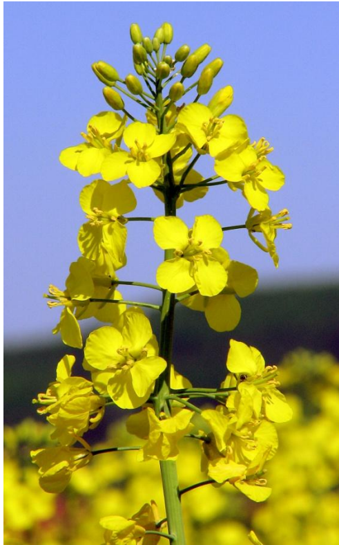
Уљана репица - Brassica napus
