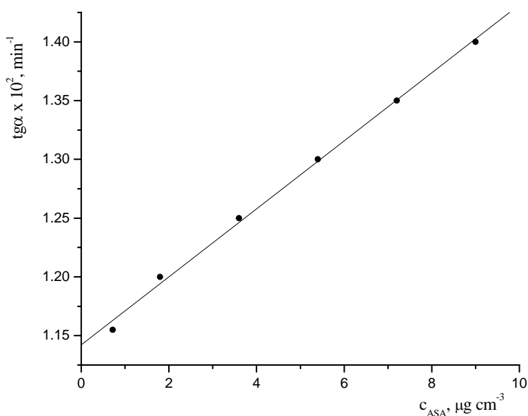
Slika 31. Zavisnost brzine reakcije od koncentracije acetilsalicilne kiseline. Koncentracije u rastvoru: c_{NaOH} = 0,1 \text{ mol dm}^{-3} , c_{R(NO)OH} = 1,5 \cdot 10^{-5} \text{ mol dm}^{-3} , c_{Co^{2+}} = 3,4 \cdot 10^{-5} \text{ mol dm}^{-3} , c_{NaCl} = 0,1 \text{ mol dm}^{-3} , t = 22,0 \pm 0,1 \text{ } ^\circ\text{C}
