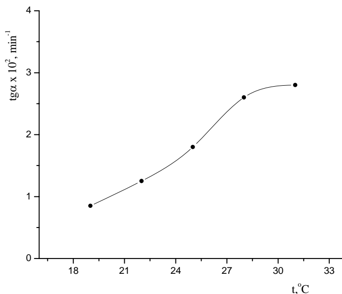
Slika 32. Zavisnost brzine reakcije od temperature. Koncentracije u rastvoru: c_{\text{NaOH}} = 0,1 \text{ mol dm}^{-3} , c_{\text{R(NO)OH}} = 1,5 \cdot 10^{-5} \text{ mol dm}^{-3} , c_{\text{Co}^{2+}} = 3,4 \cdot 10^{-5} \text{ mol dm}^{-3} , c_{\text{ASA}} = 3,0 \cdot 10^{-5} \text{ mol dm}^{-3} , c_{\text{NaCl}} = 0,1 \text{ mol dm}^{-3}
