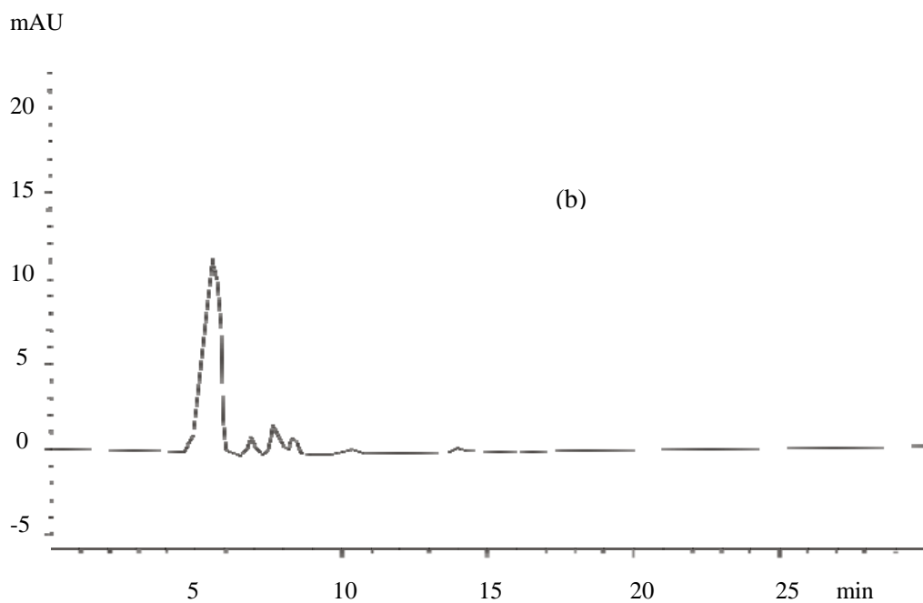
Slika 46. HPLC hromatogrami: (a) IB tablete ( 1,03 \mu\text{g cm}^{-3} ), (b) spajkovan serum ( 0,52 \mu\text{g cm}^{-3} IB). Kolona: C_{18} (Zorbax, 5\mu\text{m} , 250 \times 4,6 \text{ mm} ). Mobilna faza: fosforna kiselina-acetonitril-voda, 0,5:340:600 (V/V/V). Detekcija: UV 214 nm.
