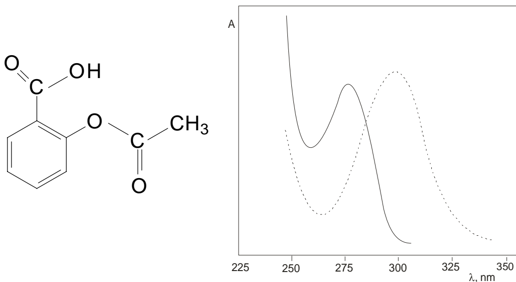
Slika 2. Hemijska struktura acetilsalicilne kiseline i UV spektar vodenog rastvora: — kisela sredina (278 nm), ... bazna sredina (298 nm)
