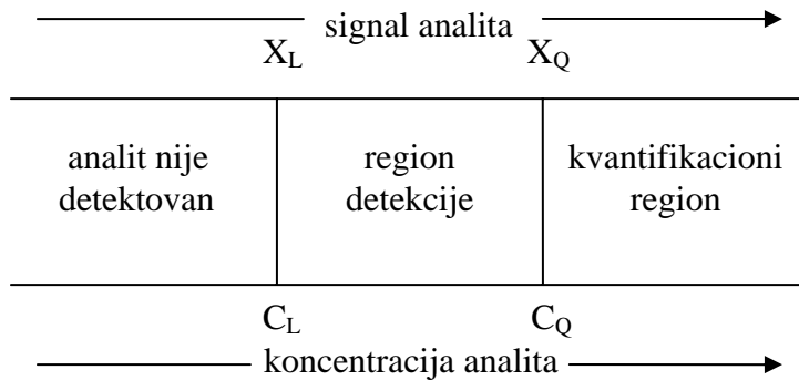
Slika 13. Regioni analitičkog određivanja
