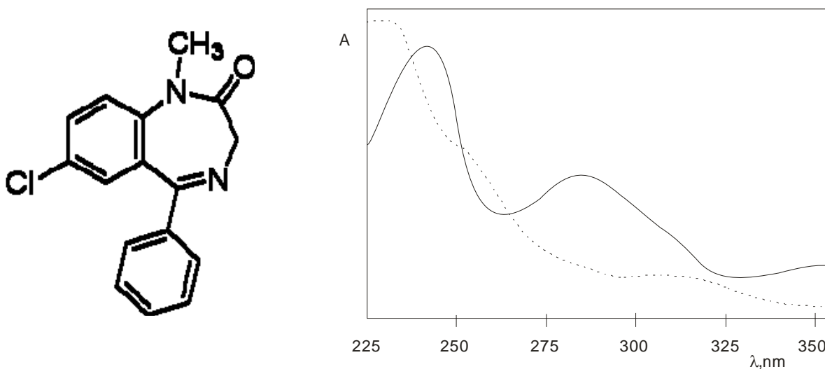
Slika 7. Hemijska struktura diazepama i UV spektar: — u vodi (kisela sredina, 242, 284, 366 nm),···· u metanolu
