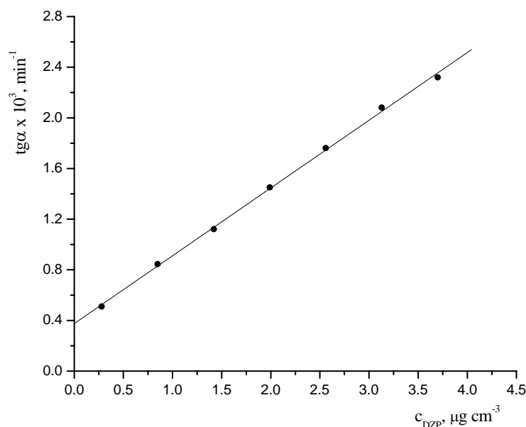
Slika 67. Zavisnost brzine reakcije od koncentracije diazepama. Koncentracije u rastvoru: c_{\text{NaOH}} = 1,5 \cdot 10^{-2} \text{ mol dm}^{-3} , c_{\text{R(NO)OH}} = 1,2 \cdot 10^{-5} \text{ mol dm}^{-3} , c_{\text{Cu}^{2+}} = 3,2 \cdot 10^{-5} \text{ mol dm}^{-3} , c_{\text{NaCl}} = 0,1 \text{ mol dm}^{-3} , t = 22,0 \pm 0,1^\circ\text{C}
