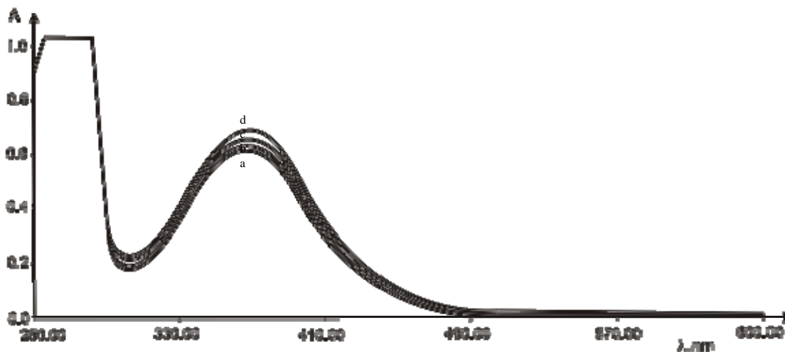
Slika 47. Promena apsorpcionog spektra 1-nitrozo-2-naftola u etanolno kiseloj sredini sa vremenom nakon dodatka dimenhidrinata: a) 1; b) 3; c) 5; d) 7 min. Koncentracije u rastvoru: c_{R(NO)OH} = 1,0 \cdot 10^{-5} \text{ mol dm}^{-3} , c_{CH_3COOH} = 0,1 \text{ mol dm}^{-3} , c_{Cd^{2+}} = 5,0 \cdot 10^{-6} \text{ mol dm}^{-3} , c_{DMH} = 1,0 \cdot 10^{-5} \text{ mol dm}^{-3}
