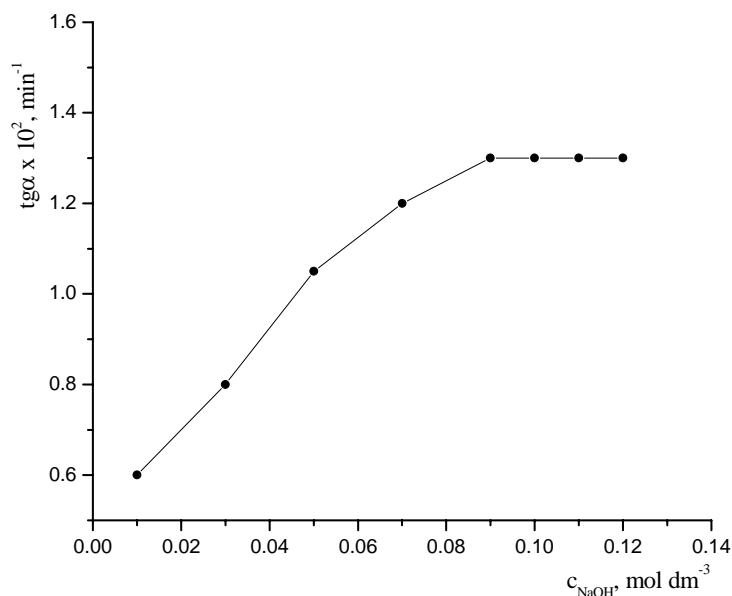
Slika 28. Zavisnost brzine reakcije od koncentracije natrijum-hidroksida. Koncentracije u rastvoru: c_{R(NO)OH} = 1,0 \cdot 10^{-5} \text{ mol dm}^{-3} , c_{Co^{2+}} = 1,7 \cdot 10^{-5} \text{ mol dm}^{-3} , c_{ASA} = 1,0 \cdot 10^{-5} \text{ mol dm}^{-3} , c_{NaCl} = 0,1 \text{ mol dm}^{-3} , t = 22,0 \pm 0,1 \text{ }^\circ\text{C}
