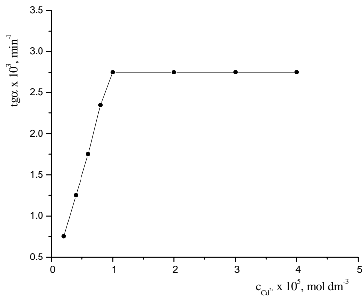
Slika 50. Zavisnost brzine reakcije od koncentracije Cd(II). Koncentracije u rastvoru: c_{CH_3COOH} = 7,0 \cdot 10^{-2} \text{ mol dm}^{-3} , c_{R(NO)OH} = 1,8 \cdot 10^{-5} \text{ mol dm}^{-3} , c_{DMH} = 1,0 \cdot 10^{-5} \text{ mol dm}^{-3} , c_{NaCl} = 0,1 \text{ mol dm}^{-3} , t = 22,0 \pm 0,1^\circ \text{C}
