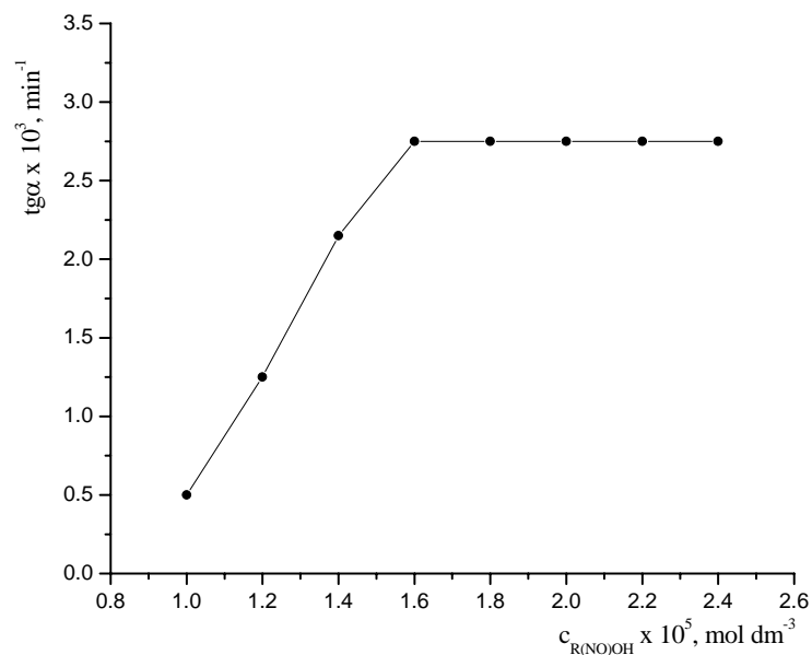
Slika 49. Zavisnost brzine reakcije od koncentracije 1-nitrozo-2-naftola. Koncentracije u rastvoru: c_{CH_3COOH} = 7,0 \cdot 10^{-2} \text{ mol dm}^{-3} , c_{Cd^{2+}} = 1,0 \cdot 10^{-5} \text{ mol dm}^{-3} , c_{DMH} = 1,0 \cdot 10^{-5} \text{ mol dm}^{-3} , c_{NaCl} = 0,1 \text{ mol dm}^{-3} , t = 22,0 \pm 0,1^\circ \text{C}
