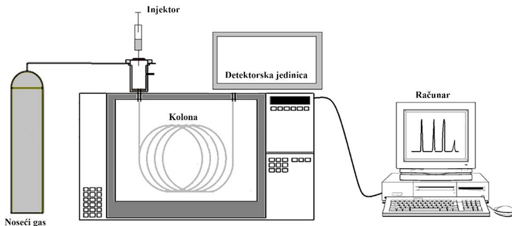
Slika 17. Šema gasnog hromatografa (Castro Vasconcellos i saradnici, 2015)
