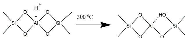
Slika 14. Termički tretman kiselinski modifikovanog zeolita na temperaturi od 300 °C
